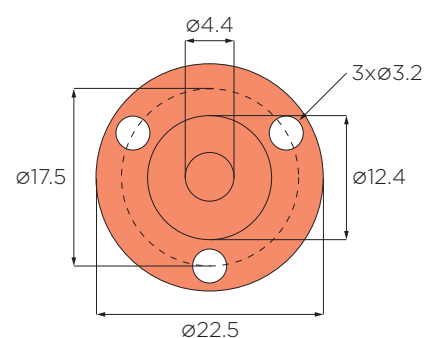
E FLANGE
