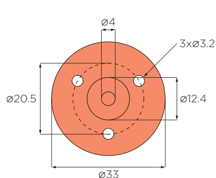
F FLANGE
